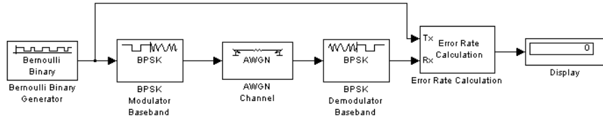
doc_bpsk
